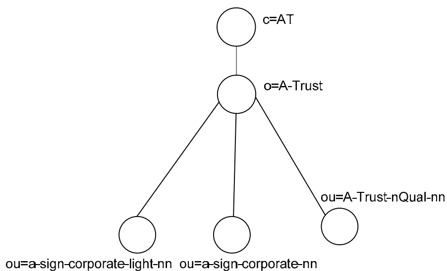
Abbildung 2 a.trust Verzeichnisbaum
